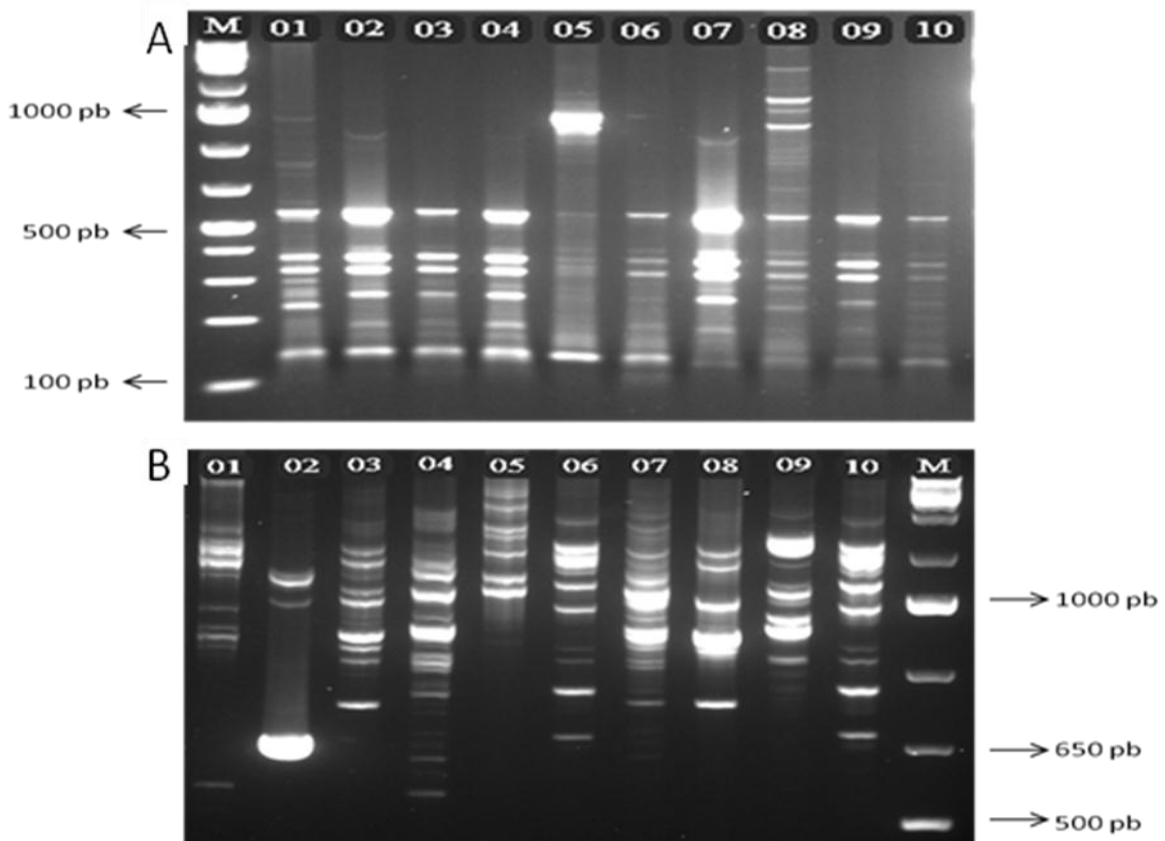
Figura 5. Em A. Perfis eletroforéticos das bandas geradas por ERIC-PCR. B. Perfis eletroforéticos das bandas geradas por BOX-PCR, onde M representa Marcador 1Kb Plus DNA Lander Fermentas e os números de 01 á 10 corresponde aos isolados M10, M16, BRS10B, BRS10A, PS11, PS6A, P2A, P15B, FH1A, e FH8 respectivamente.
