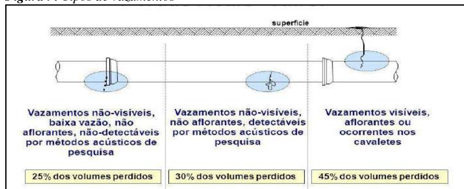
Figura 9: Tipos de vazamentos
